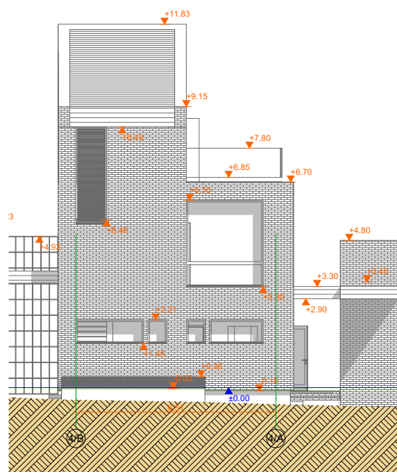
4N_D 1:100
