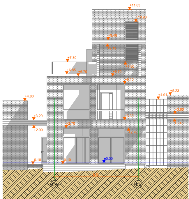
4N_B 1:100
