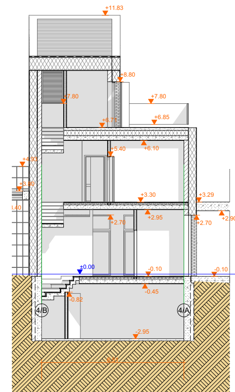
4B Pjūvis 1:100
