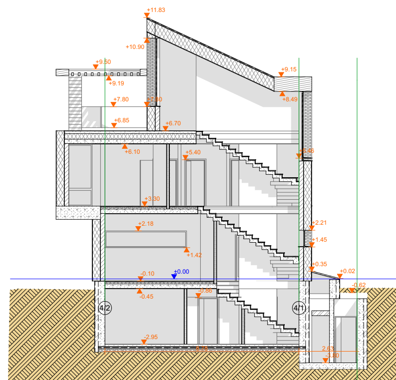
4A Pjūvis 1:100
