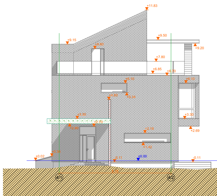
4N_C 1:100
