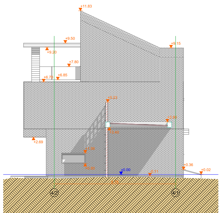
4N_A 1:100
